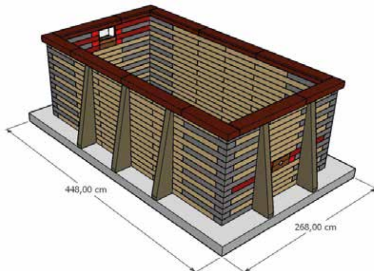
POSE HORS-SOL/SEMI-ENTERRÉE (1/3 ENTERRÉE) 10X RENFORTS OBLIGATOIRES
